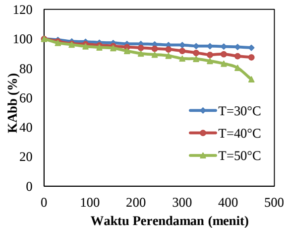
Gambar 8. Grafik pengaruh suhu perendaman terhadap rasio kadar air dengan konsentrasi 30,7 °Brix.
